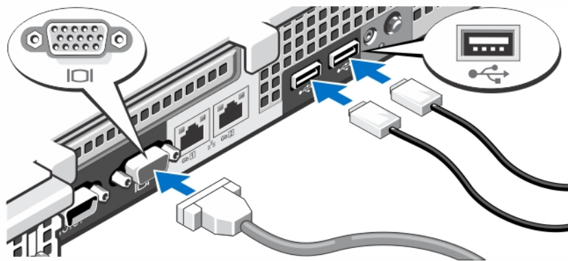
그림 2. 선택 사항 — 키보드, 마우스 및 모니터 연결
