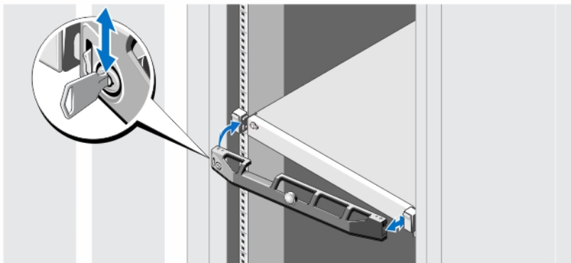
그림 6. 베젤(선택 사항) 설치
